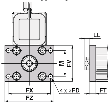
Mặt bích trực: LEY32□□B-□□□F 25 40 A C
