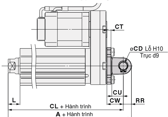
Gá chữ U: LEY32□□B-□□□D 25 40 A C
