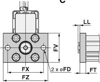
Mặt bích trực: LEY32□□B-□□□F 25 40 A C
