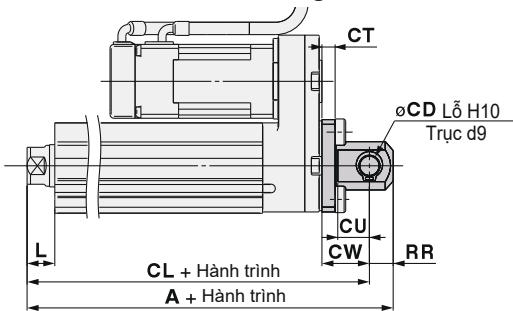
Gá chữ U: LEY32□□B-□□□D 25 40 A C
