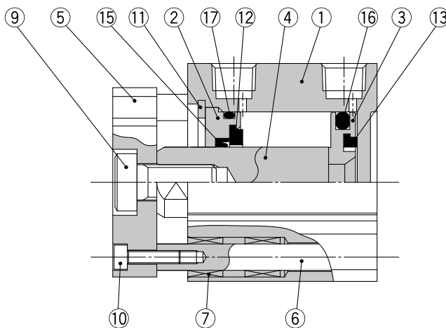
Dòng xylanh kèm cảm biến (Có vòng từ bên trong thân)
