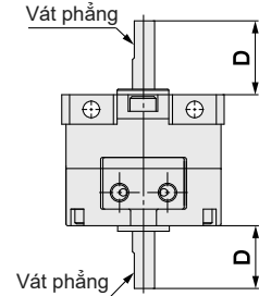
2 Trục/CRBU2Y
