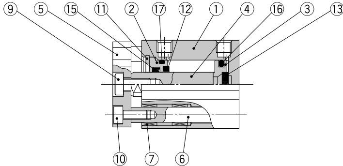
Dòng xylanh kèm cảm biến (Có vòng từ bên trong thân)
