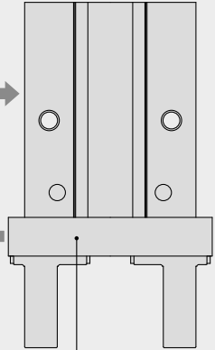
Thanh trượt dẫn hướng Kích thước nòng 20 mm
